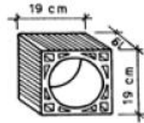
BLOK BACA TUĞLALARI
