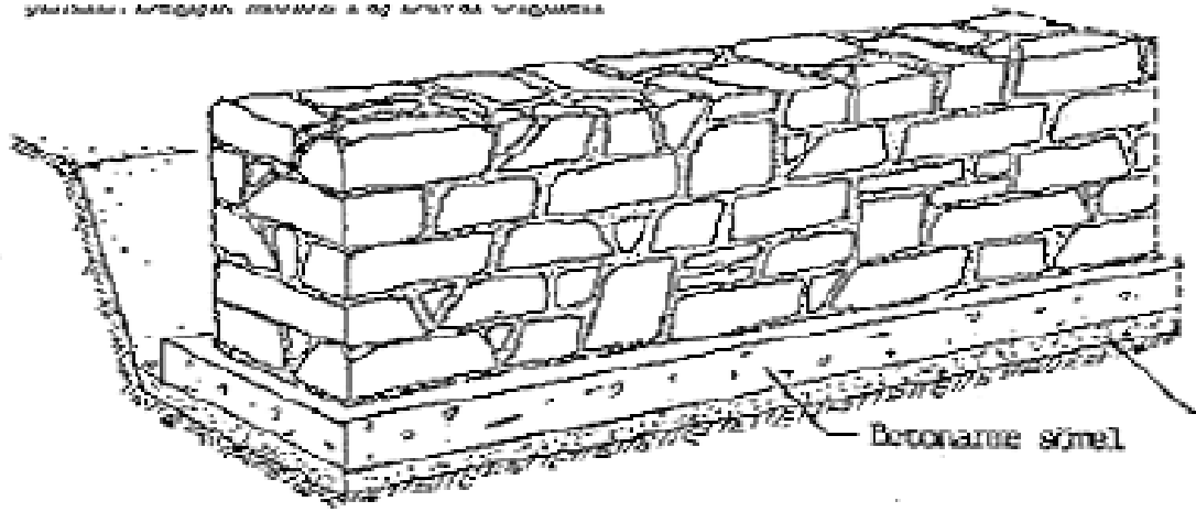
Yatay Derzli Moloz Taş Duvar
