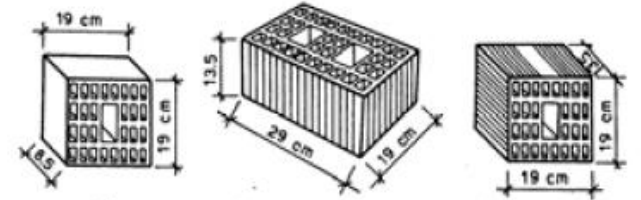
DÜŞEY DELİKLİ TAŞIYICI BLOK TUĞLALAR
