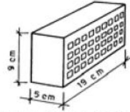
DELİKLİ MAKİNA TUĞLASI (NORMAL TUĞLA)
